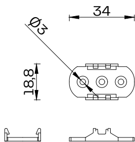
Clip (Scale 1:2)
