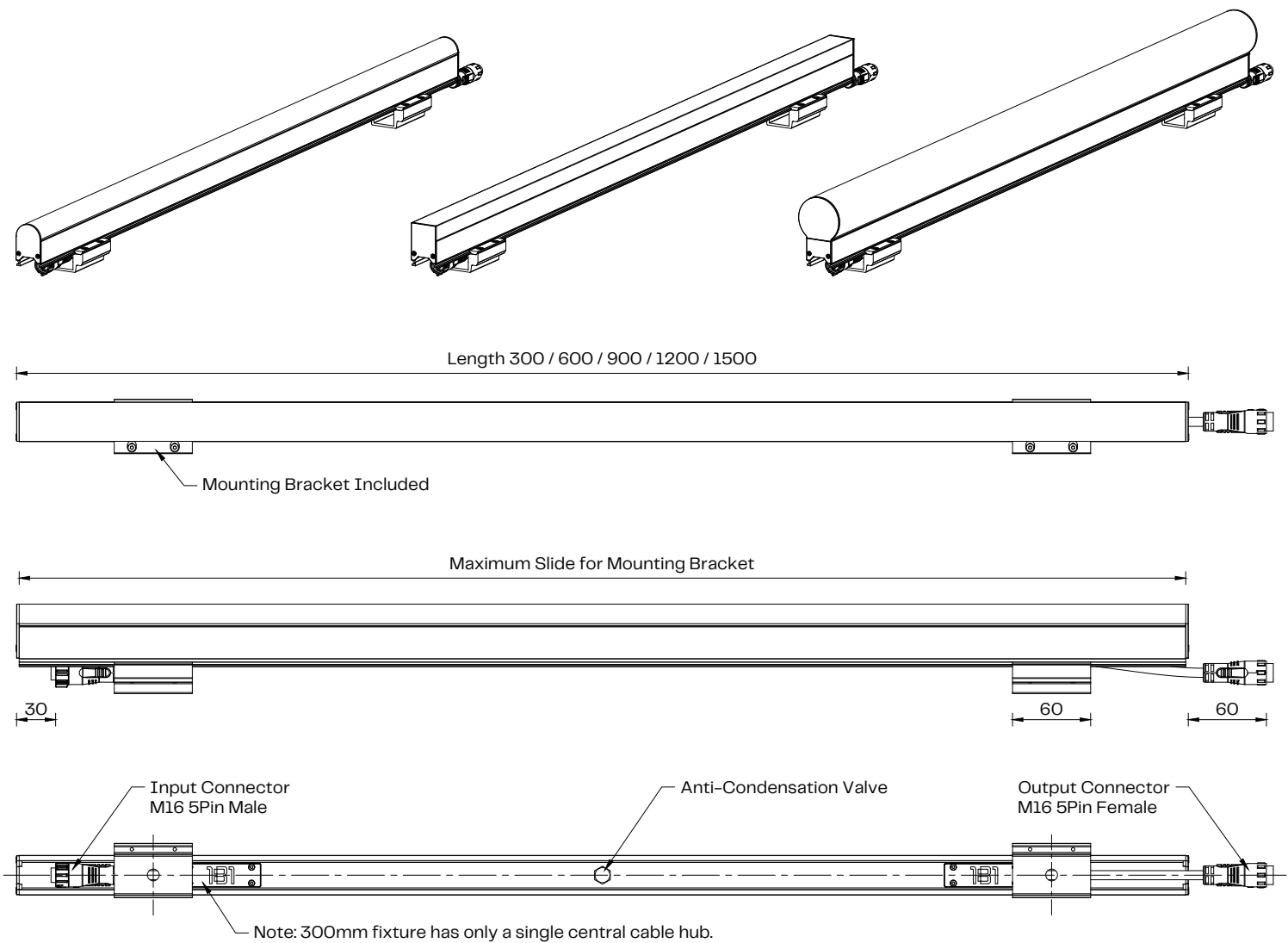
DiGi Linear E-Series 2 Scale 1:5
